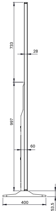
СХЕМА ДИСПЛЕЯ (ВИД СЛЕВА)
