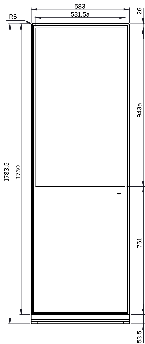
СХЕМА ДИСПЛЕЯ (ВИД СПЕРЕДИ)
